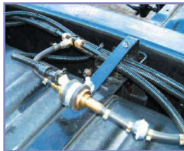
Figur 7a (venstre) & 7b – placering af samling ved indsprøjtningsted
