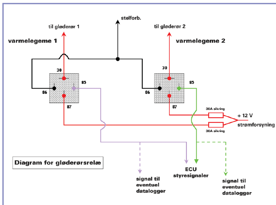
Figur 1 Viser relædiagram for gløderør.
